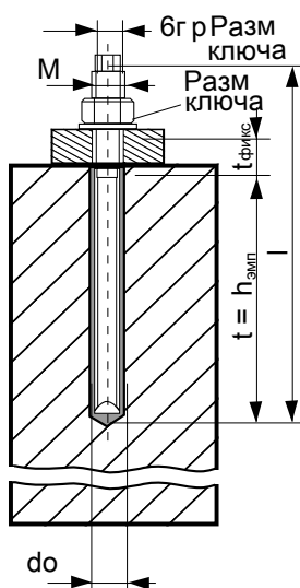
Рис. 5: Размеры
