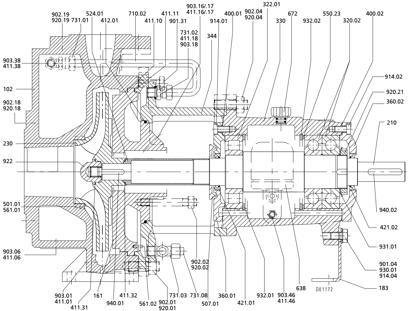
Рис. 19: Сборочный чертеж
