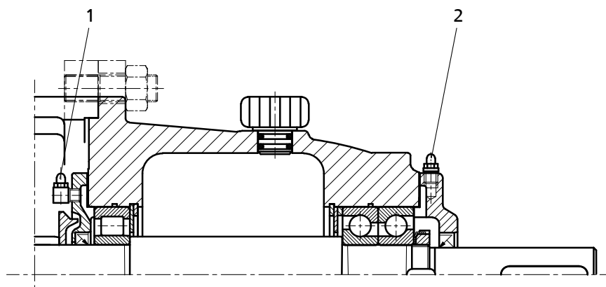
Рис. 16: Положение смазочных ниппелей
