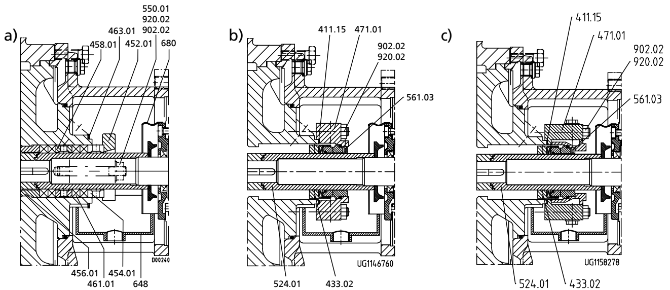
Рис. 20: Исполнение с сальниковой набивкой (а), торцевым уплотнением с цилиндрической крышкой корпуса (b), торцевым уплотнением с обогреваемой крышкой корпуса (с)
