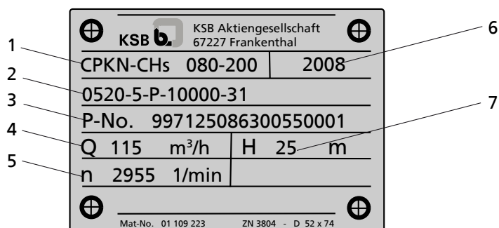
Рис. 5: Заводская табличка (пример)
