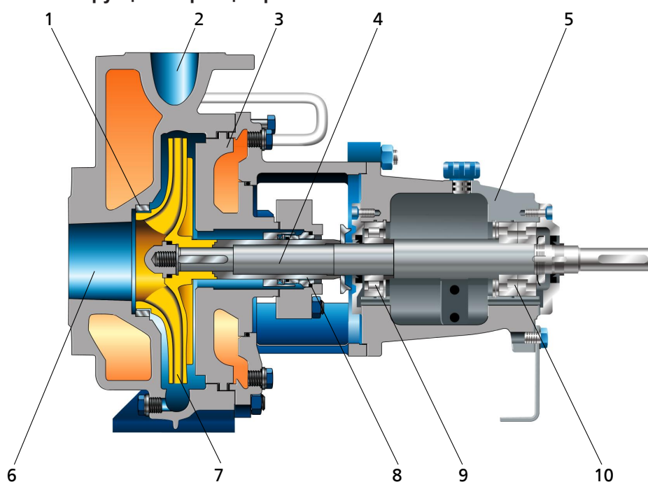
Рис. 6: Сечение
