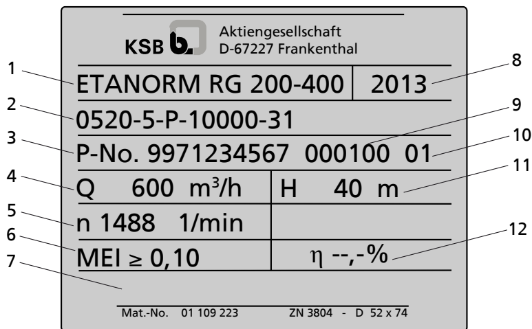
Рис. 5: Заводская табличка (пример) Etanorm-R
