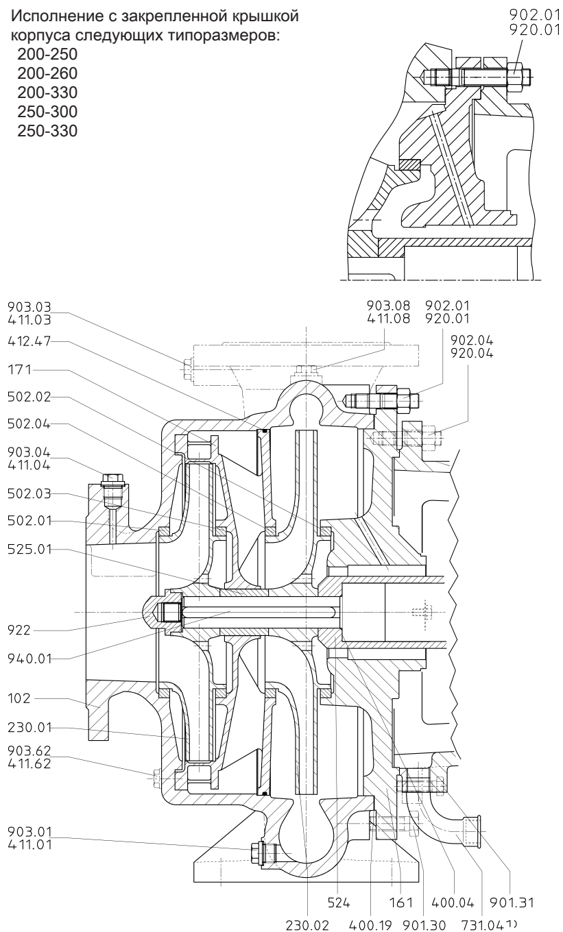
Рис. 30: Типоразмер 125-500/2 (двухступенчатый)
