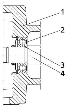
Рис. 18: Монтаж радиальных шарикоподшипников
