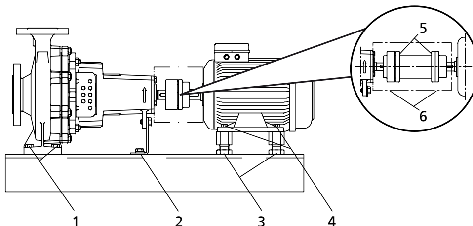
Рис. 24: Позиции затяжки винтов насосного агрегата
