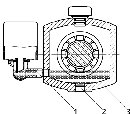
Рис. 17: Корпус подшипников с регулятором уровня масла
