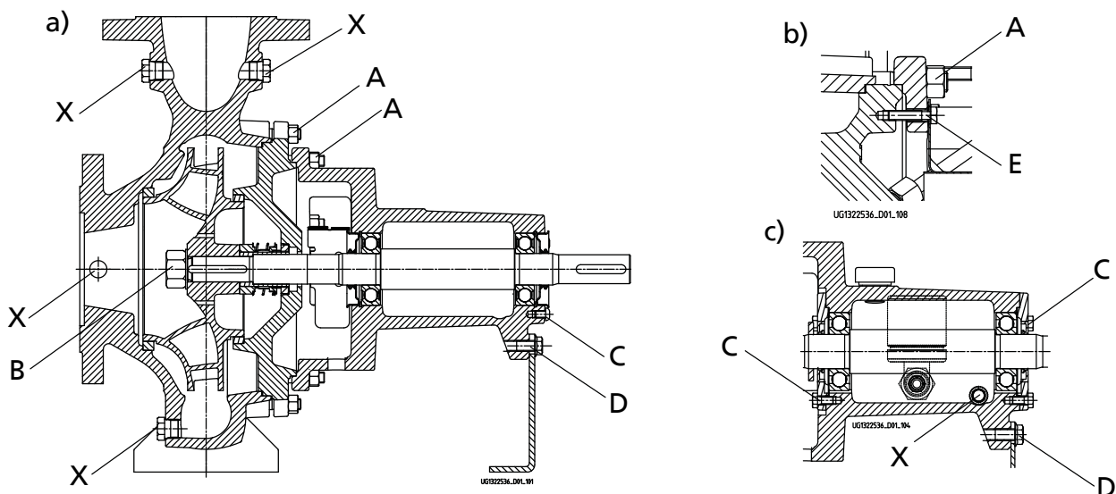
Рис. 23: Места затяжки резьбовых соединений: исполнение с привинчиваемой крышкой корпуса и консистентной смазкой (a), исполнение с зажимной крышкой корпуса (b) и смазкой жидкой смазкой (c)
