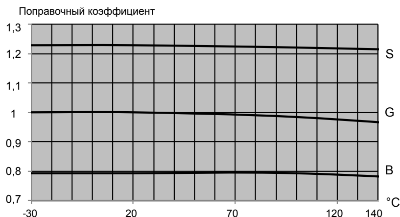
Рис. 11: Диаграмма температурной коррекции для материала корпуса G (JL1040/ A48CL35B), S (JS1030/A536 GR 60-40-18) и B (CC480K-GS/B30 C90700)
