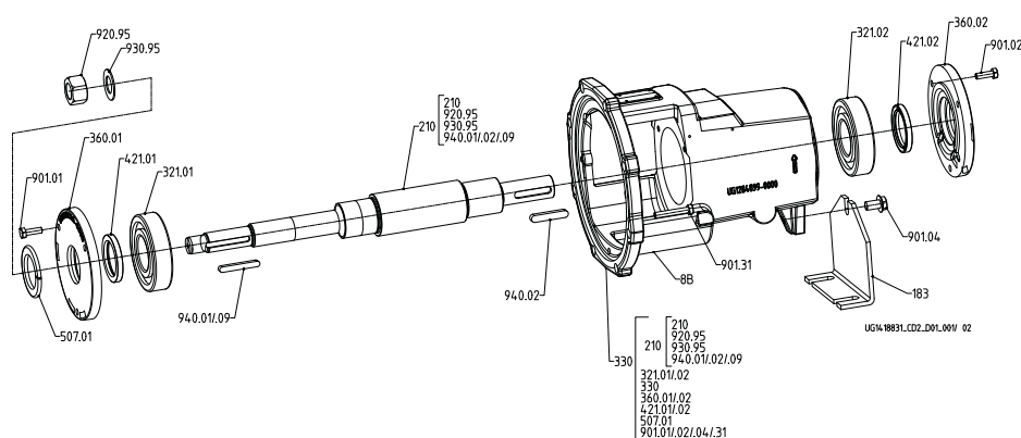
Рис. 29: Исполнение с усиленным подшипниковым узлом (узел вала 50 и 60)
