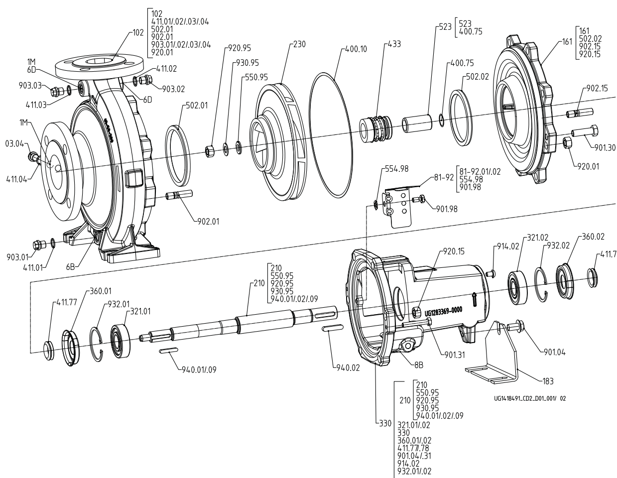
Рис. 25: Исполнение со стандартным торцевым уплотнением и привинчиваемой крышкой корпуса
