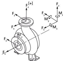
Рис. 10: Силы и моменты на патрубках насоса
